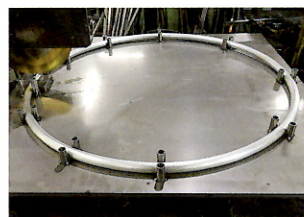
テーブル 天板フレーム アルミ異径材φ25(リブ付)、 リング径φ700mm
