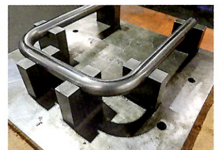
自動車シートフレーム STKM 13A φ19.1mm、曲げ35R
