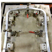
レセプションチェアのフレーム アルミ□19mm、曲げ7カ所、 溶接6カ所
