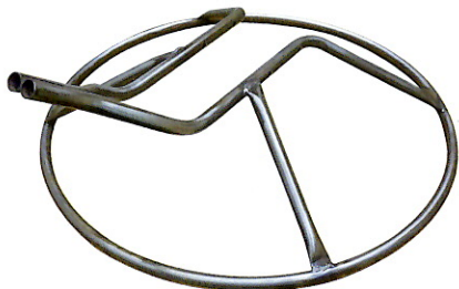
コンクリートならしフレーム スチールφ19.1mm、リング径400mm、溶接14カ所
