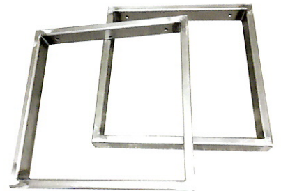
テーブル脚 スチール□50x20mm 完成品サイズL680x580mm、溶接16カ所
